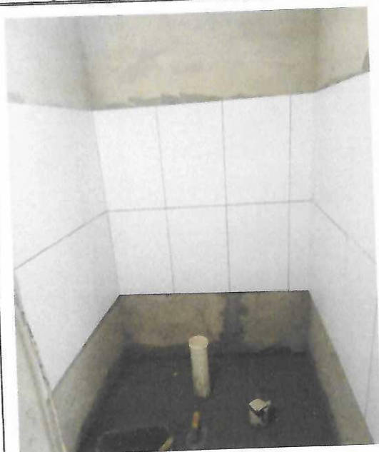
Imagem 03 – Revestimento ceramico para parede, 15 x 15 cm, azulejo branco, tipo "A", aplicado com argamassa industrializada ac-i, rejuntado, exclusive emboço - Bloco Vestiário de Times.
