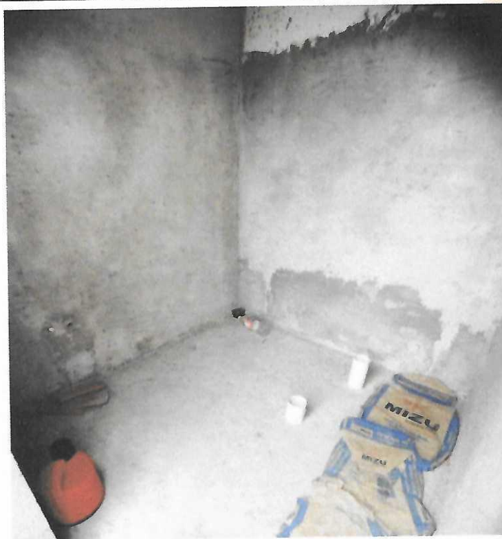
Imagem 20 - Ponto de água fria embutido, c/material pvc rígido soldável Ø 25 mm - Bloco Camarote.
