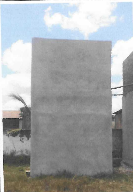
Imagem 17 - Reboco especial de parede 2cm com argamassa traço t1 - 1:3 (cimento / areia) - Fosso da Caixa d'água.
